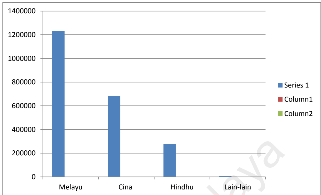
Rajah 1.3: Jumlah Penduduk Mengikut Kumpulan Etnik Di Luar Bandar, Negeri Perak, 2010.
